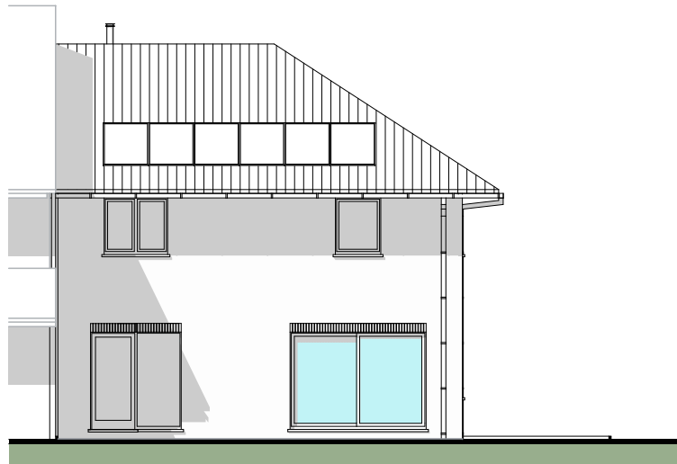
ACHTERGEVEL
