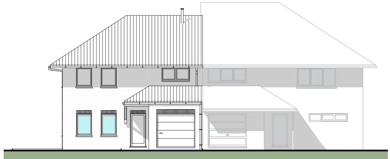
VOORGEVEL
