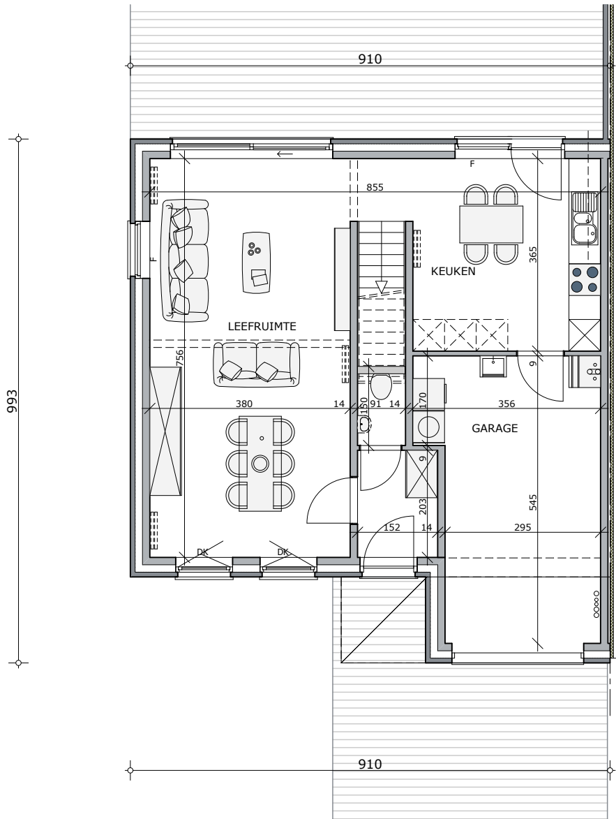
GELIJKVLOERS Opp.= 81.04 m 2
